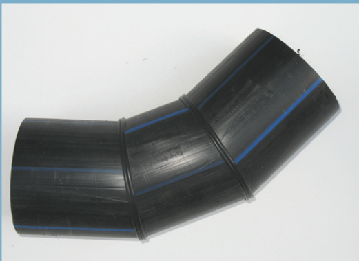
Luk 45° od polietilena PE 100 dimenzija od 63-315 mm
